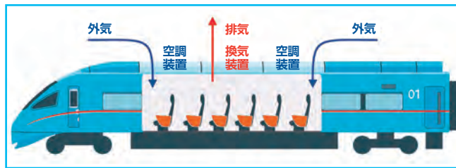
ロマンスカーの換気の仕組み
