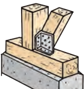
筋かいプレート設置
