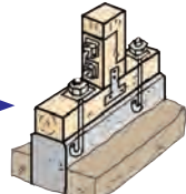
腐食した土台と柱を取り替え、金物で固定
