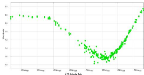
ベテルギウスの変光過程
