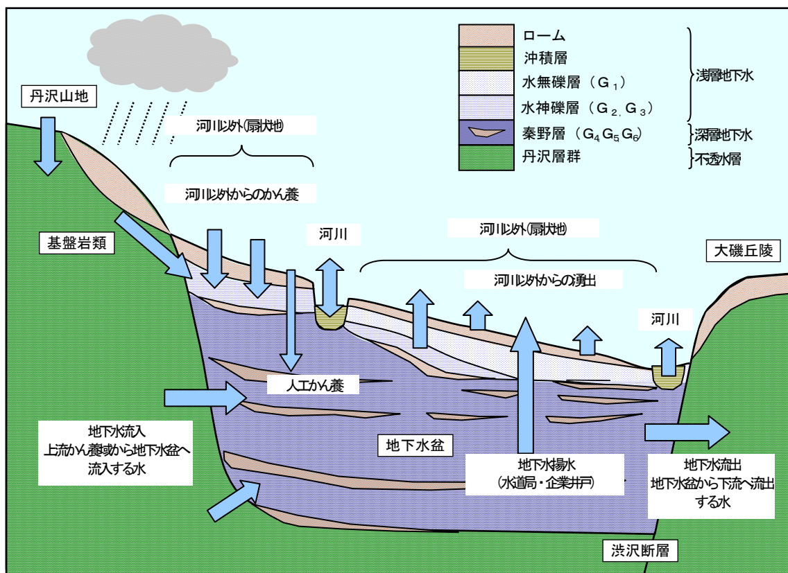
図 1-6 地域水循環
