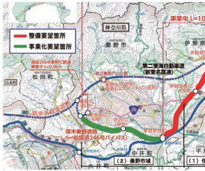
厚木秦野道路(国道246号バイパス)計画図
