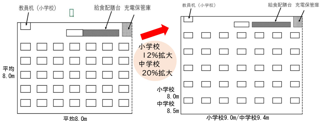
図3-2 普通教室の拡大
