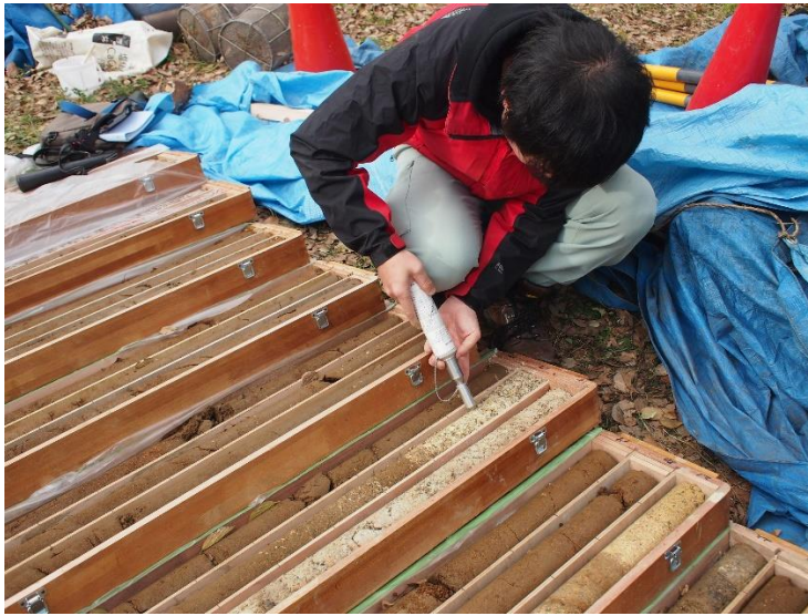
ボーリング資料の針貫入試験
