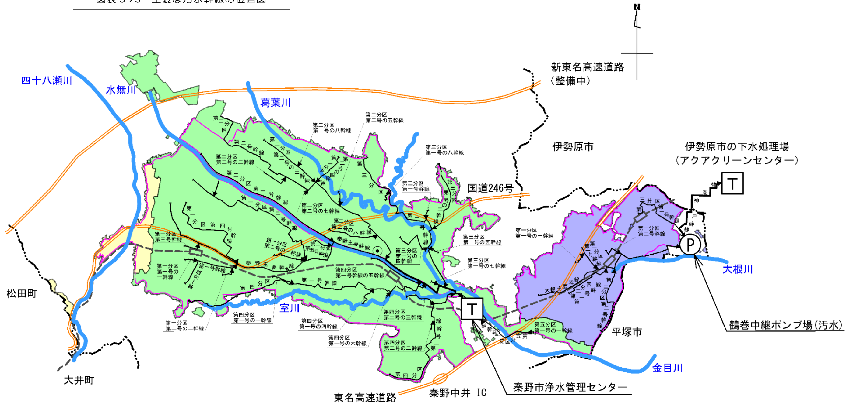
図表 3-25 主要な汚水幹線の位置図
