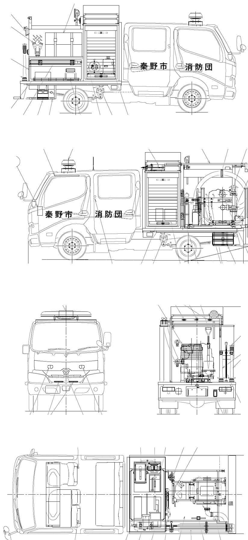
消防団用小型動力ポンプ付積載車概要図
